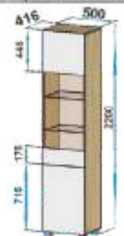
Пенал со стеклом
