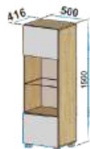
Шкаф низкий со стеклом
